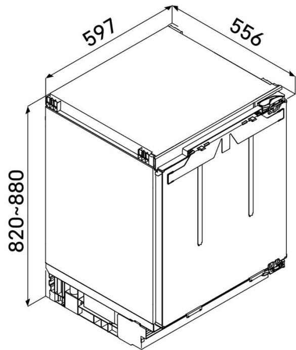
製品本体寸法（縦横高さ）
