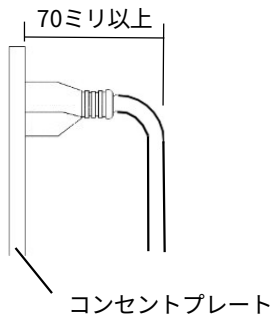
パナソニック電工 品番：WN1131（相当品）
