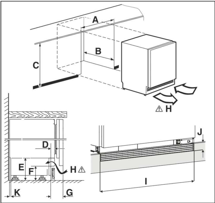
設置時の有効寸法
