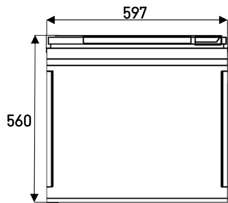
製品本体寸法（天面図）
