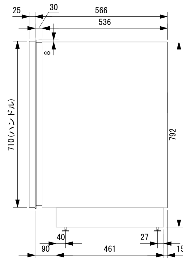
側面図
