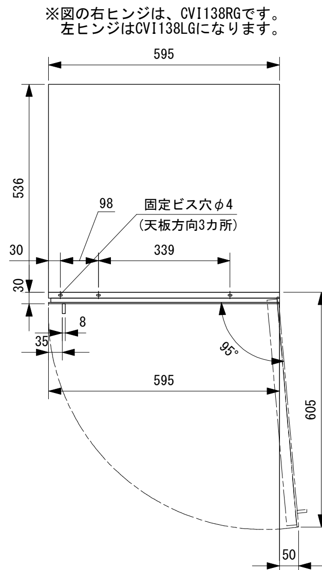
平面図
