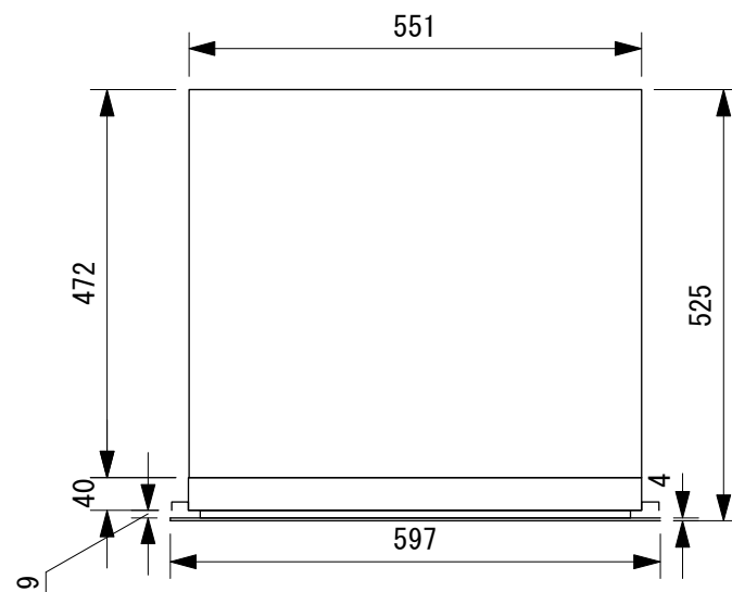
平面図
