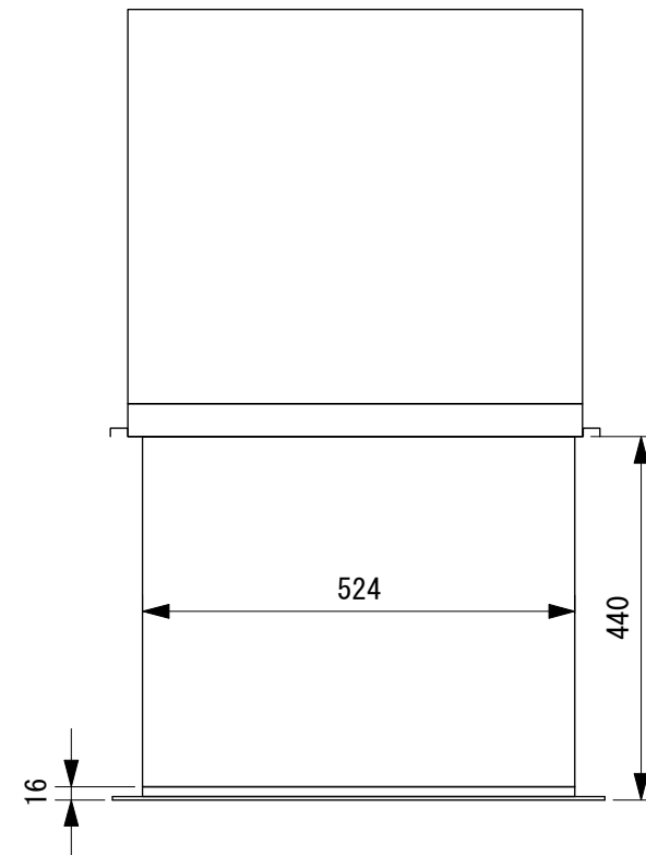
側面図
