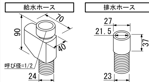
ホース類
