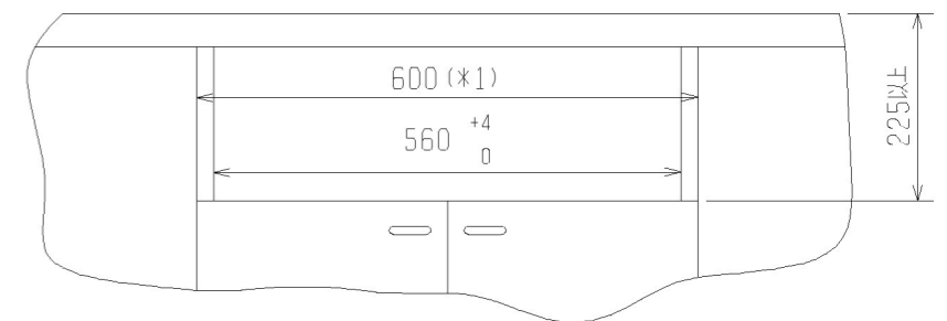
【取り付け穴】
