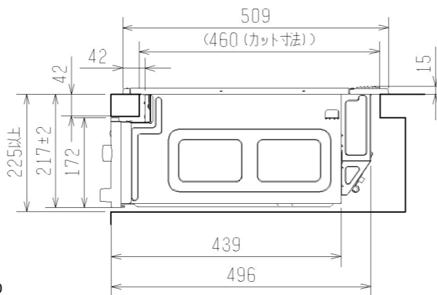
【側面図】
