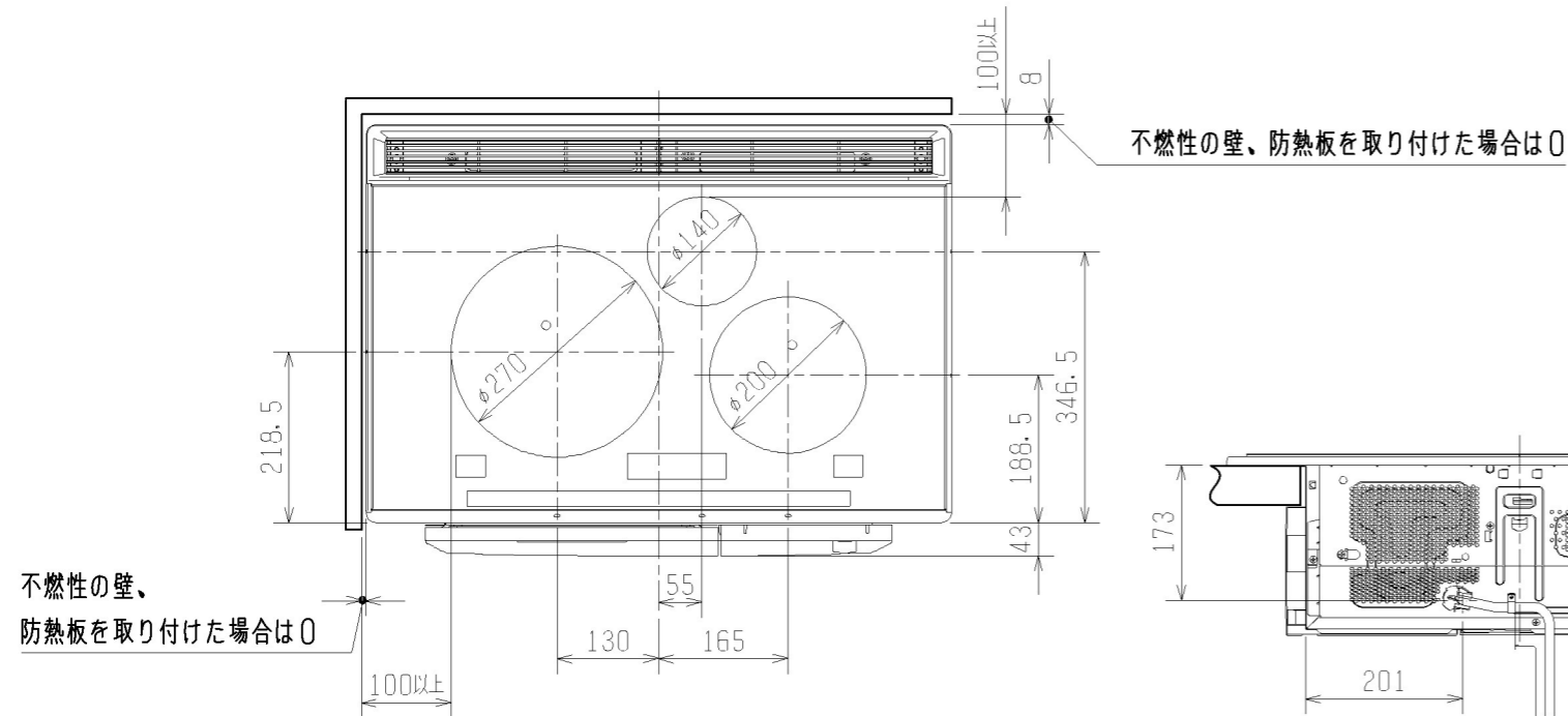
【上面図】
