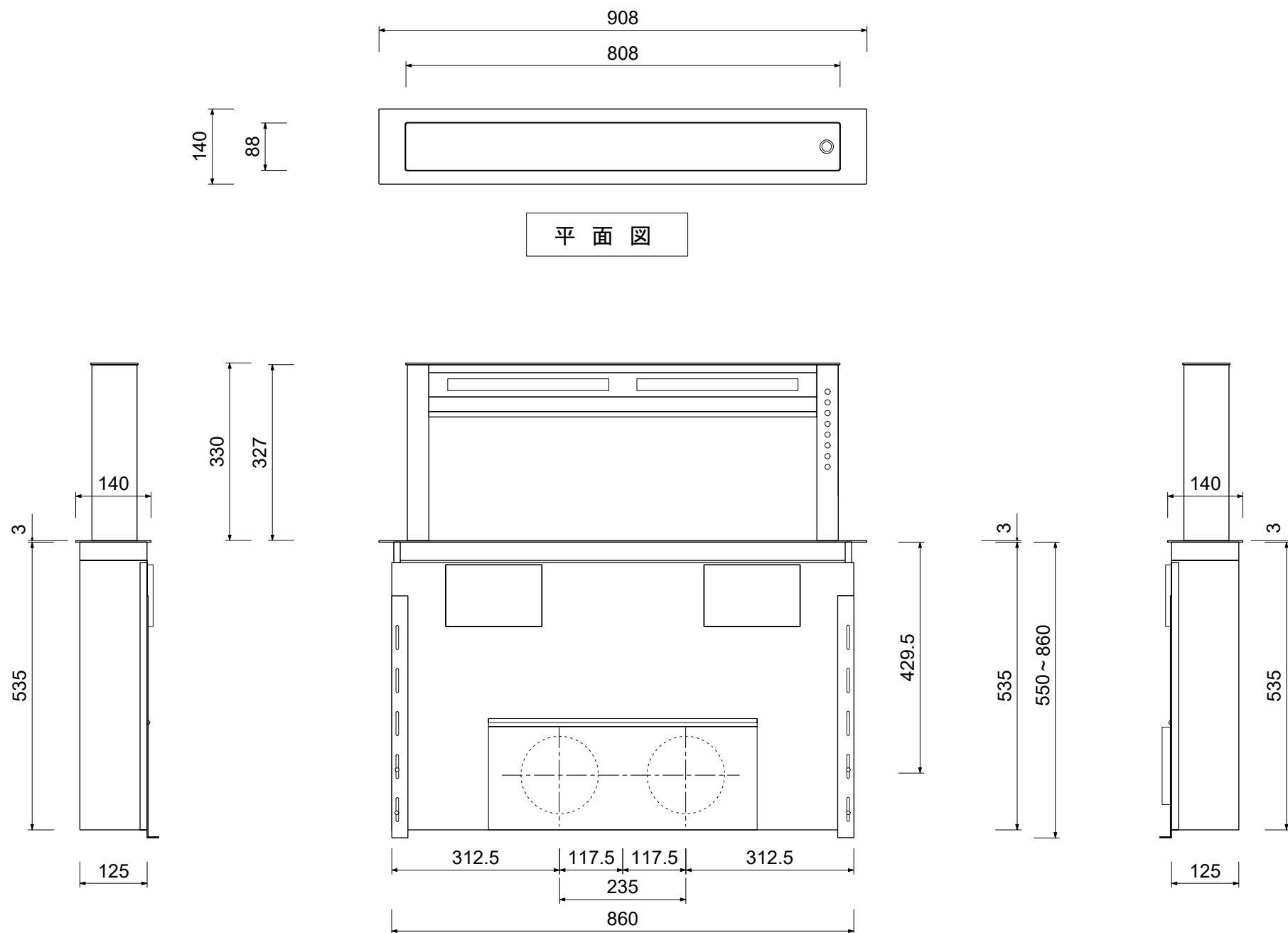
側面図
