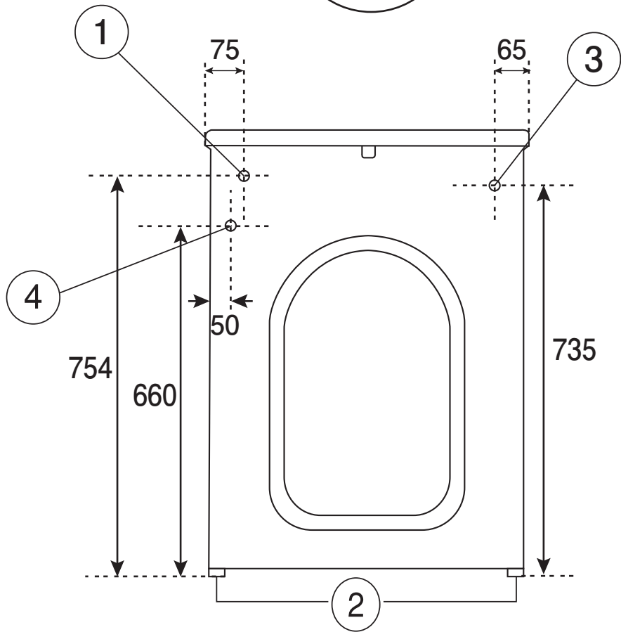
背面図
