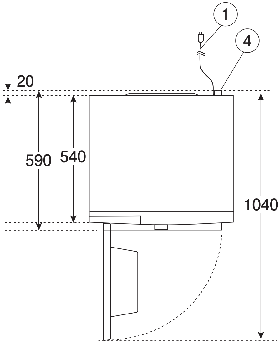
上面図
