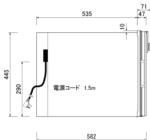
左側面図
