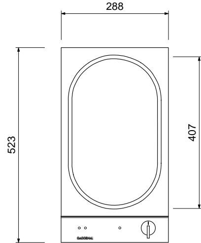
上面図
